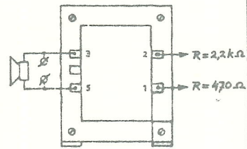
GELUID UITGANGS TRAFU SOUND OUTPUT TRANSF. TONAUSC. ÜBERTRAGER 50 051 581
