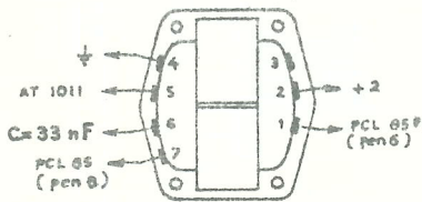
RASTERUITGANGS TRAFU FRAME OUTPUT TRANSF. BILDAUSC. ÜBERTRAGER AT 3507 50 051 708
